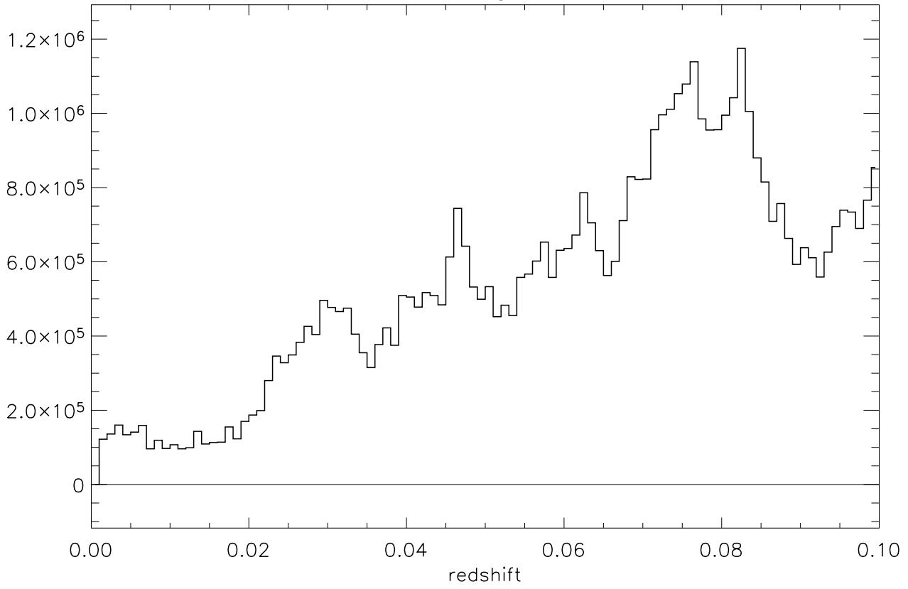
all SDSS galaxies
